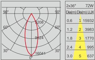
R71 2x36W 4000K 36°
