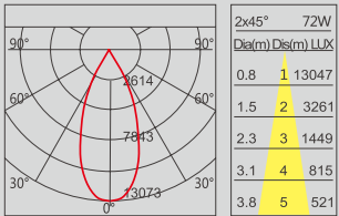
R86 2x36W 4000K 45°
