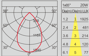
R34 20W 4000K 65°
