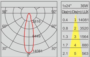
R70 36W 4000K 24°
