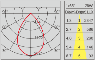
R83 26W 4000K 65°
